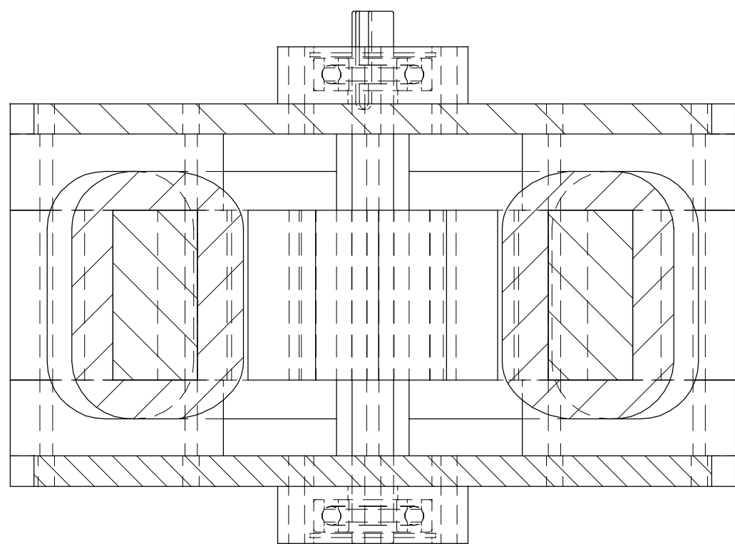
Schnitt B-B
